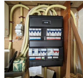
Foto 6: Groepenkast
