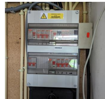
Foto 7: Groepenkast
